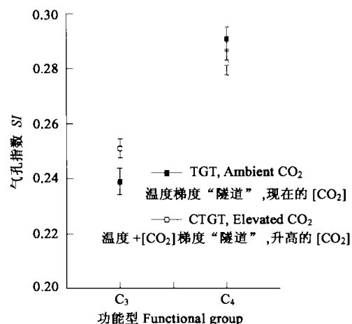
图4 C 3 和C 4 两个功能型的SI对[CO 2 ]变化的响应
