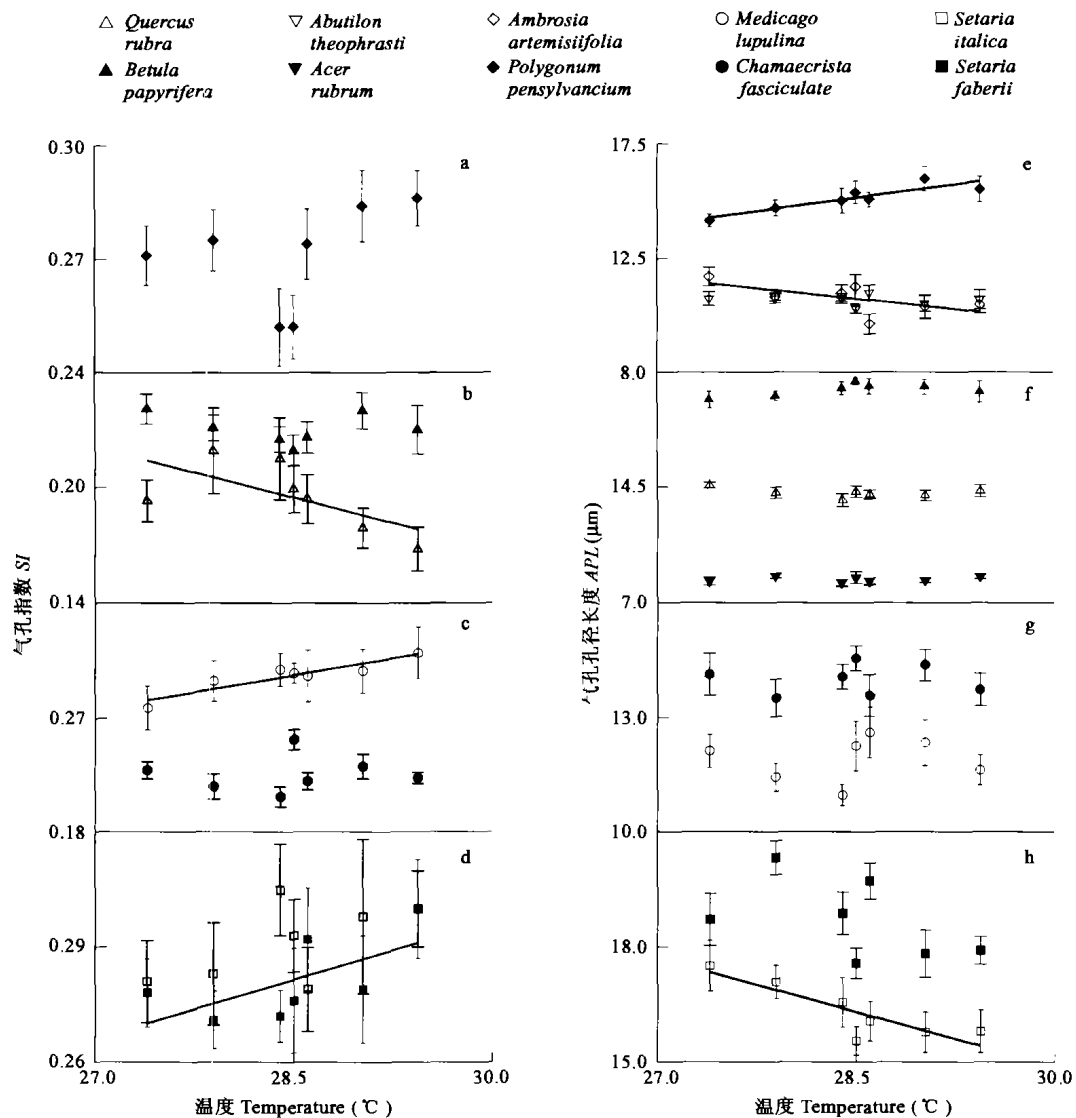
图 2 SI 和 APL 沿温度梯度的变化趋势
