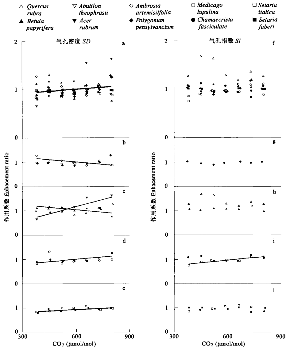
图1 \text{CO}_2 对于 SD 和 SI 的作用系数
