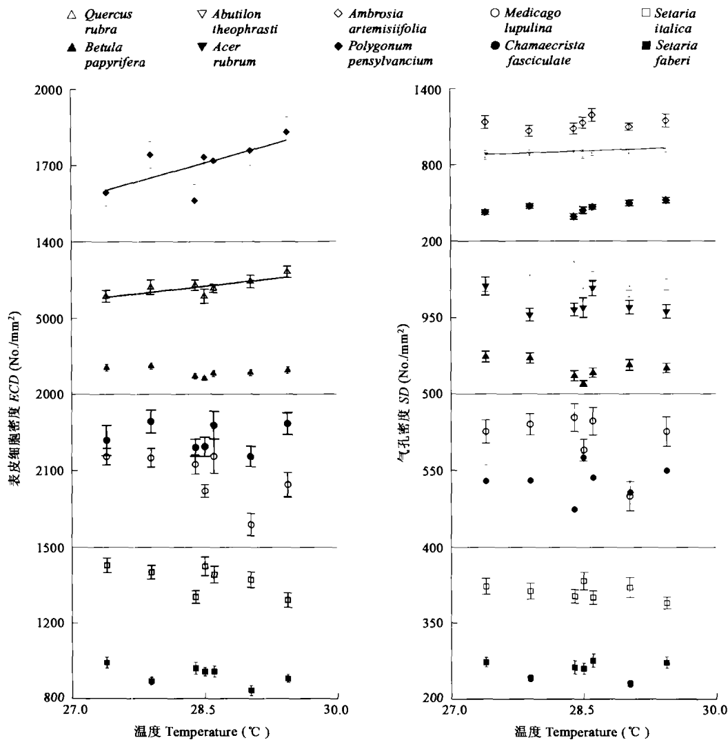
图3 ECD 和 SD 沿温度梯度的变化趋势
